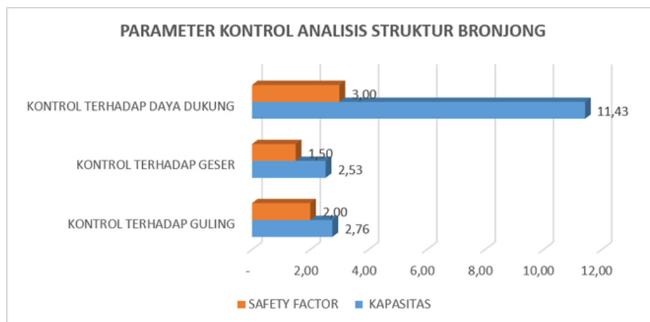
Gambar 4. Kontrol Analisis Struktur Bronjong
